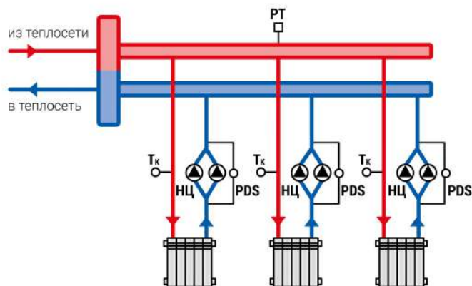
Рисунок 4.4 – Схема трех прямых контуров отопления
