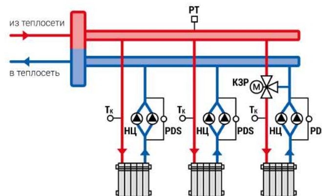
Рисунок 4.2 – Схема смесительного и двух прямых контуров отопления
