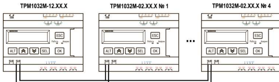
Рисунок 6.16 – Подключение TPM1032M-02.XX.X к TPM1032–12.XX.X
