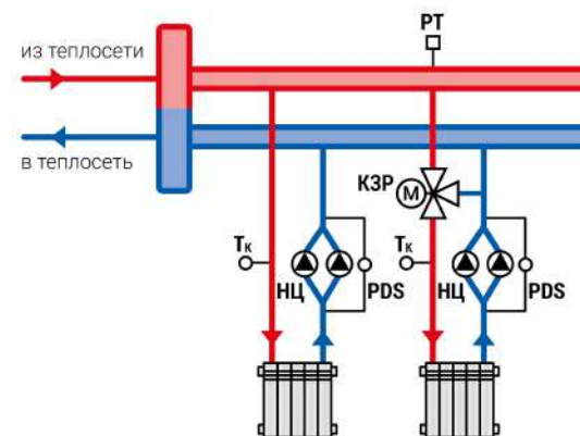
Рисунок 4.1 – Схема смесительного и прямого контура отопления
